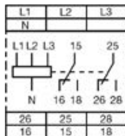
CM-MPS.11 Y 21
