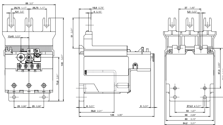
TF140DU
