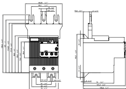
EF146-150
