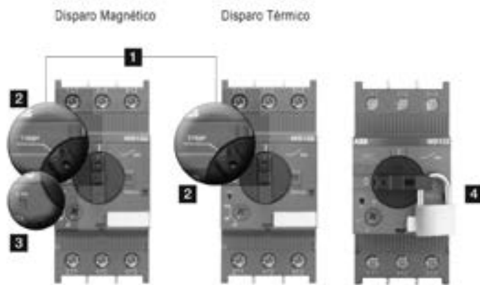
Iniciación disparo
