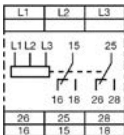
CM-MPS.31 Y 41
