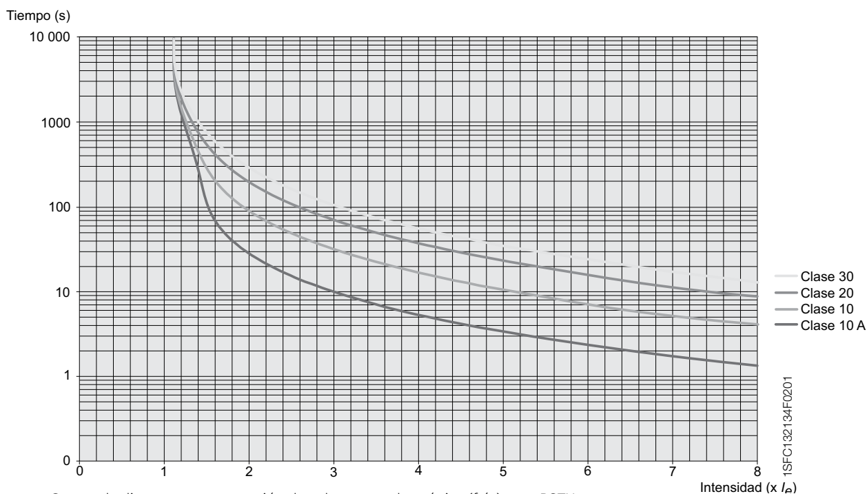
Curvas de disparo para protección de sobrecarga electrónica (frío) para PSTX.
