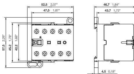
B6, B7
