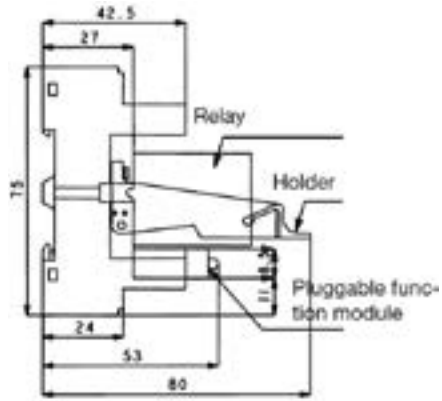
Base P/relevador CR-M
