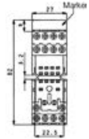
4 C/O
