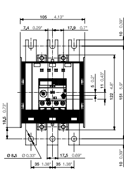
EF205-210
