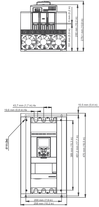
PSTX210 ... PSTX370
