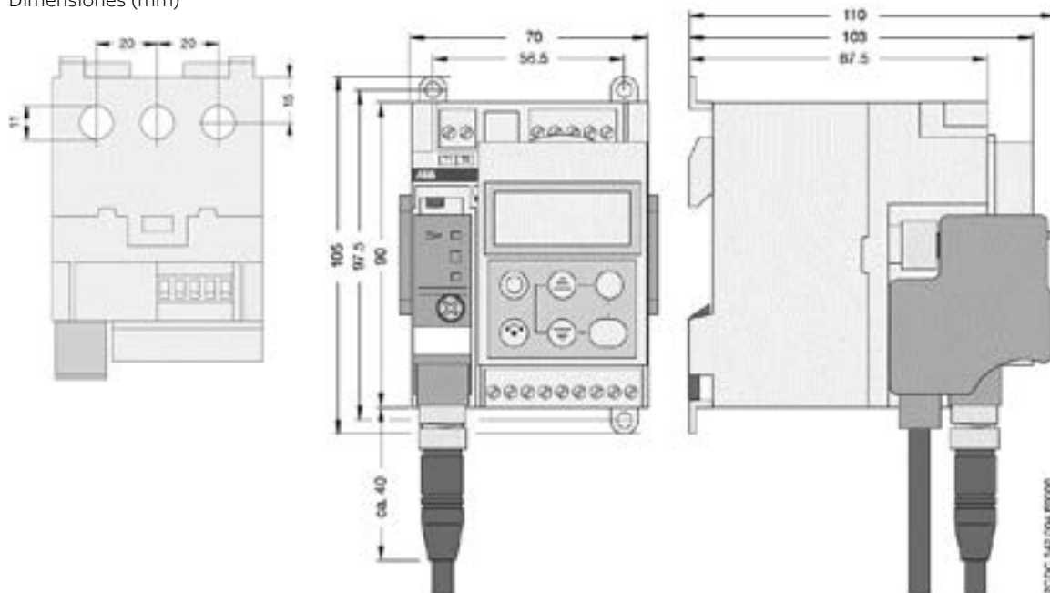
Dimensiones (mm)
