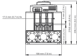
PSTX142 ... PSTX170
