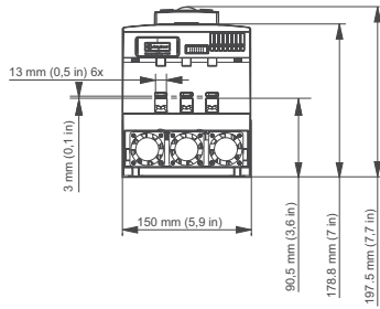
PSTX30 ... PSTX105
