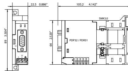
PDP32, PDR31
