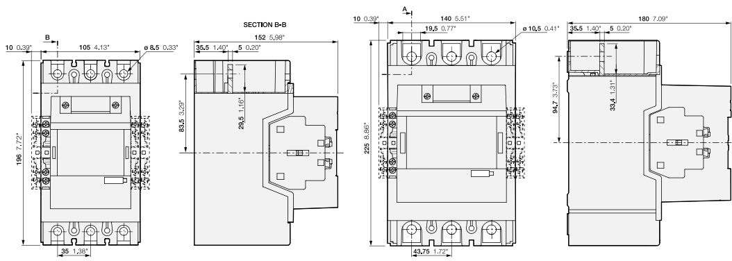
AF190, AF205
