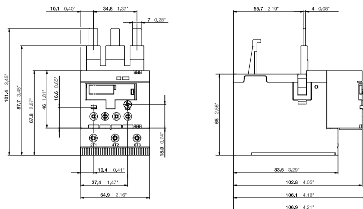
TF65
