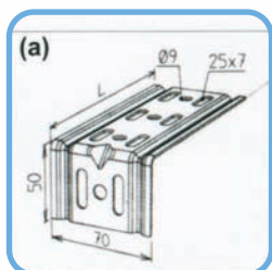
Ménsula económica
