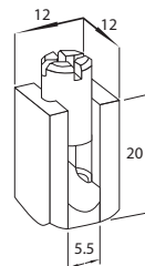
PUESTA A TIERRA MG-51-946
