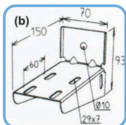
Ménsula económica reforzada
