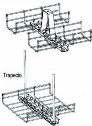
Sujetador con soporte doble
