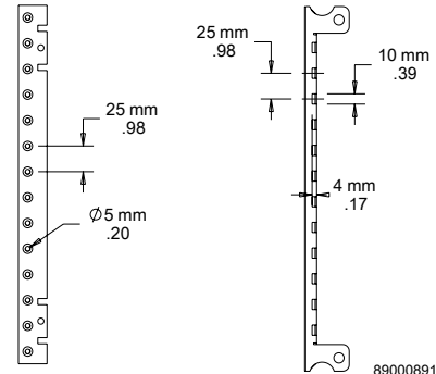
Riel delantero
