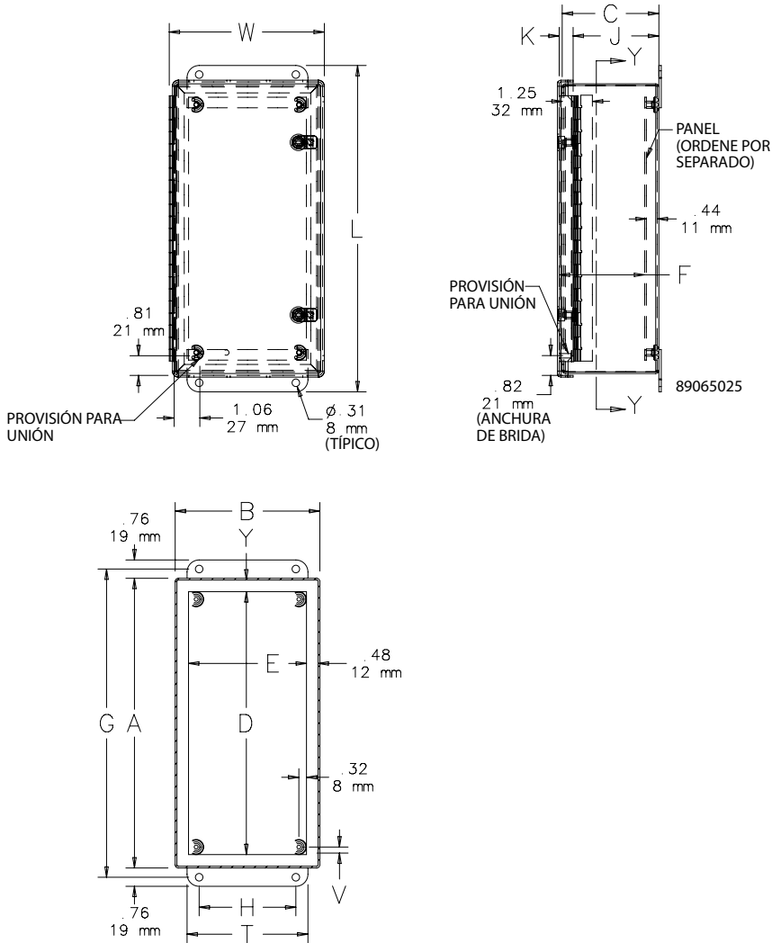
SECCIÓN Y-Y
